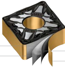
Fig.: Layer structure TTG
